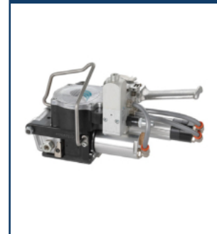
Flejadora ITI - 12
